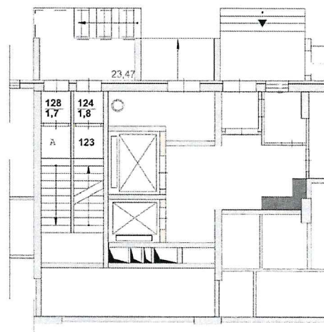
план после реконструкции
