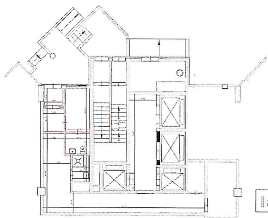
план до реконструкции
